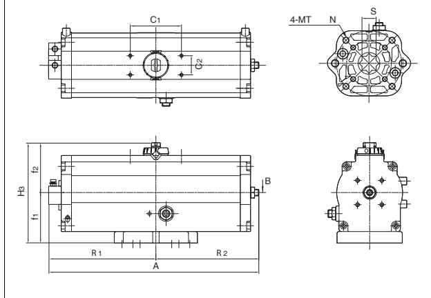
复动气缸
