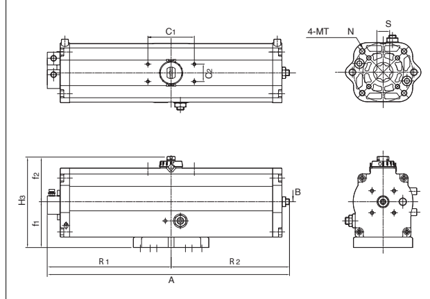
单动气缸
